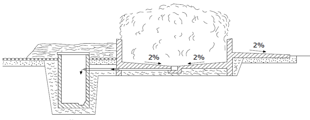
Skicë orientuese për ndërtimin e depos së plehut të ngurtë
